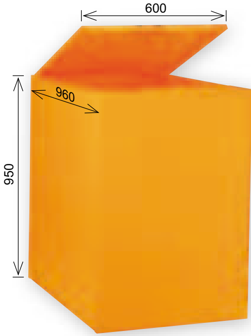
cod. 096004X0 rezervor peleŢi 350 litri
